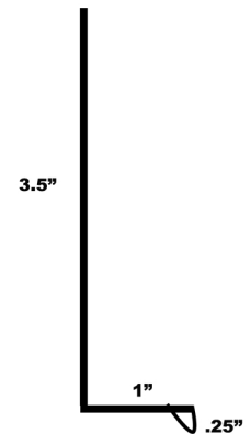
L-Wall Base
